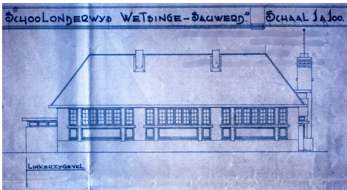
Linker aanzicht (zuidkant) volgens de oorspronkelijke bouwtekening (1936). Deze gevel zou later geheel verdwijnen achter de verbouwingen t.b.v. de winkel.
